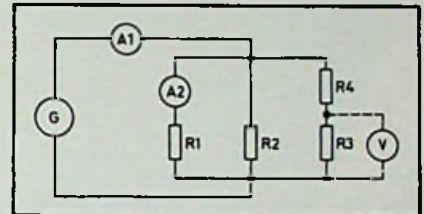
Bild 21. Prinzip der Strommessung: Strommesser A1 zeigt den Gesamtstrom durch die Schaltung an; A2 mißt den Strom durch R1. Der Strom durch R3 wird indirekt über den Spannungsabfall gemessen (Verfasser)
