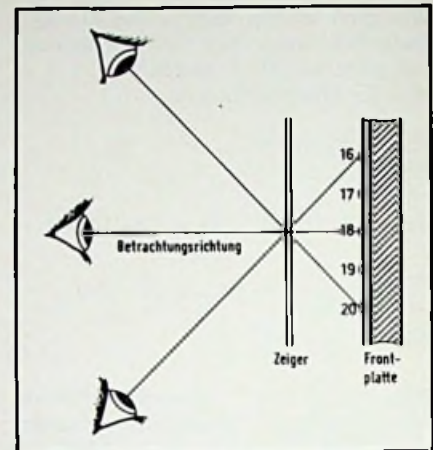
Bild 19. So entstehen bei seitlicher Ablesung eines Meßgerätes Parallaxefehler (Nordmende)
