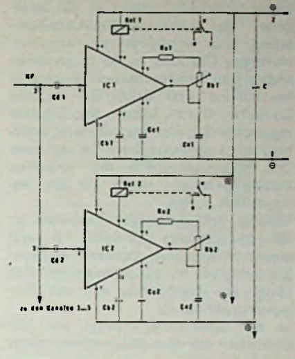
Bild 7. Schaltbild der Schaltstufen einer Tonfrequenzanlage
