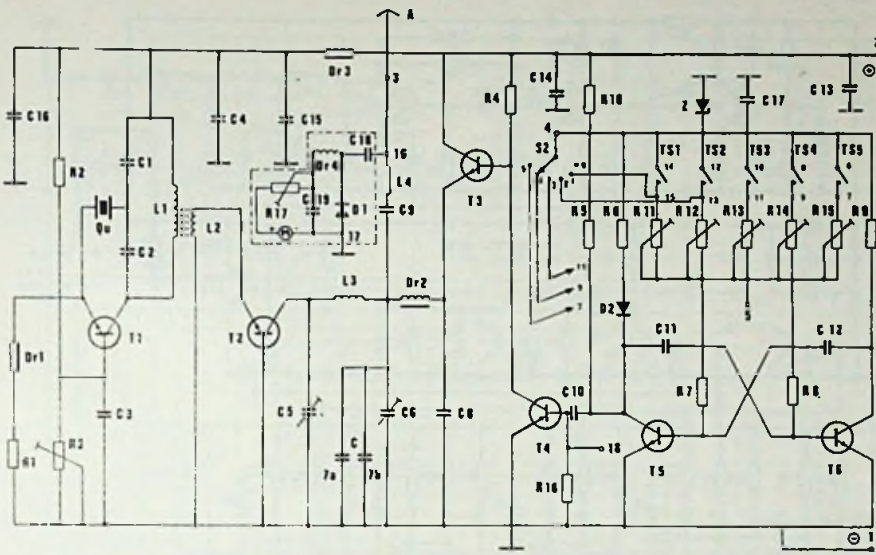
Bild 5. Schaltbild des Senders einer Tonfrequenzanlage
