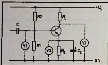
Bild 25. Meßpunkte einer Transistorstufe (Verfasser)
