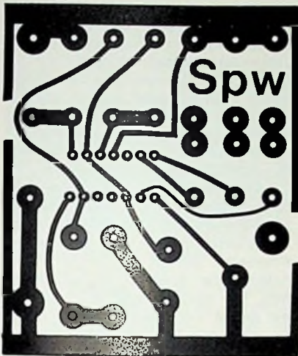
Platine im Maßstab 1:1
