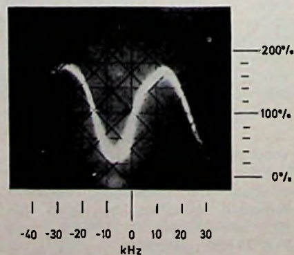
Bild 5. Bildschirmkurve einer starken Reflexion mit kleinem Umweg
