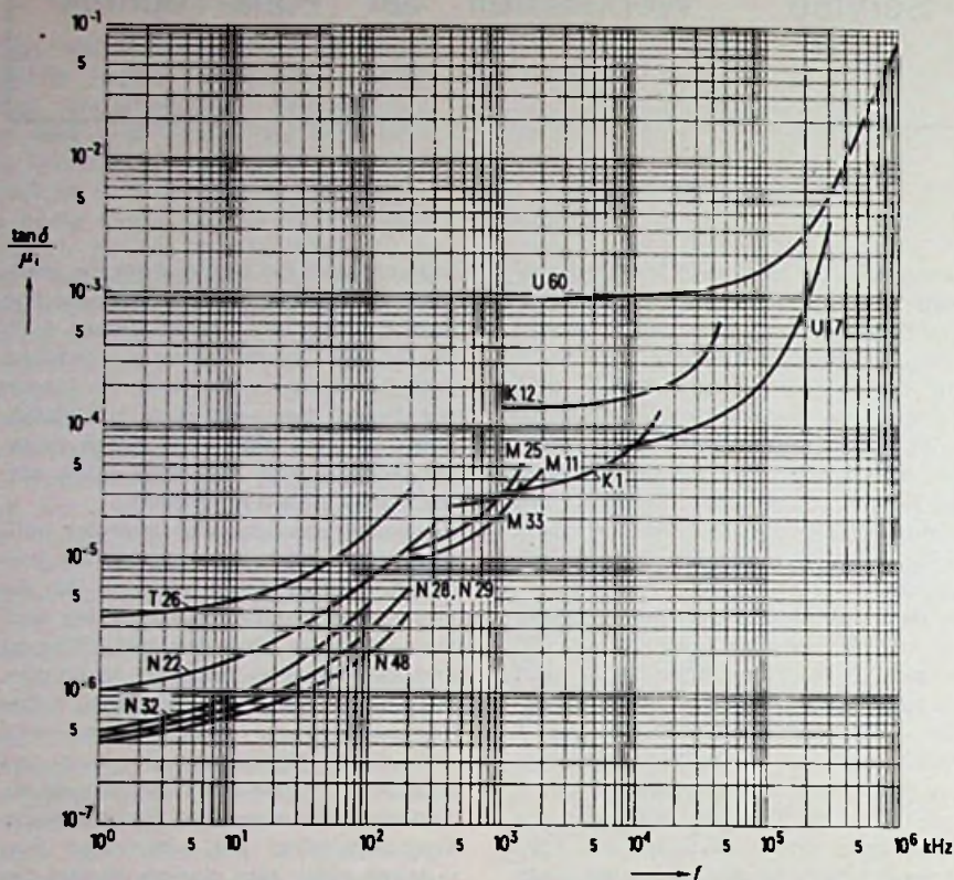
Abmessungen der Probekerne: D_A = 10 \text{ mm} , d_i = 6 \text{ mm} , h = 4 \text{ mm} Meßinduktion B \leq 1 \text{ mT}
