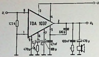
Mit bemerkenswert wenig externen Bauteilen ist dieser NF-Verstärker aufgebaut
