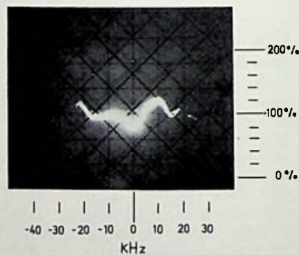
Bild 4. Bildschirmkurve einer schwachen Reflexion mit großem Umweg
